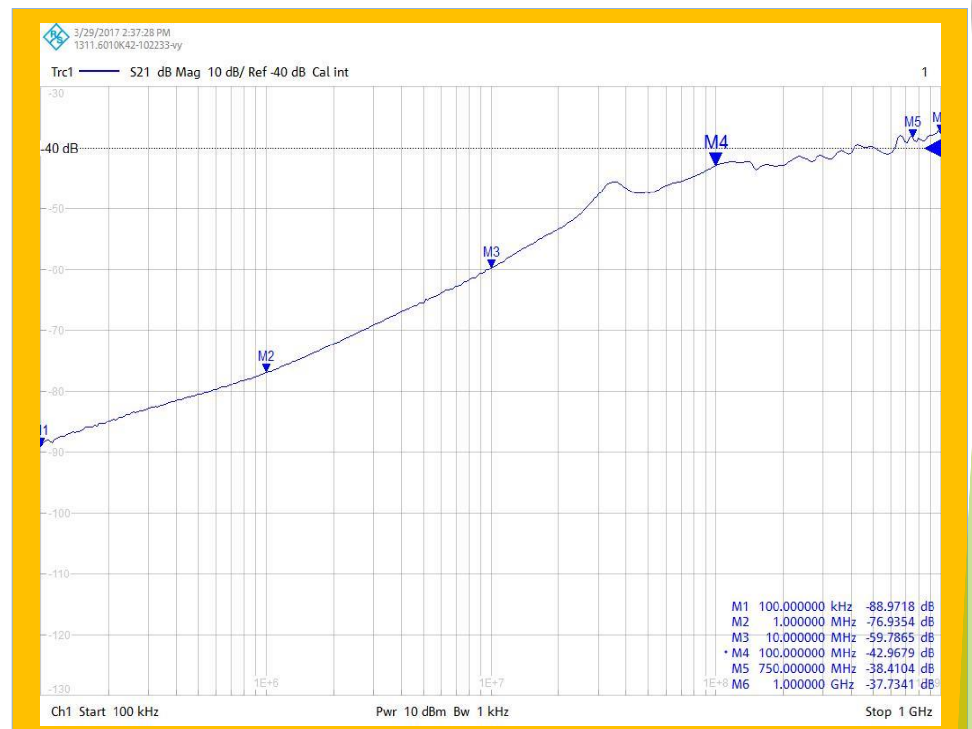
MT-871周波数特性(3軸とも)
