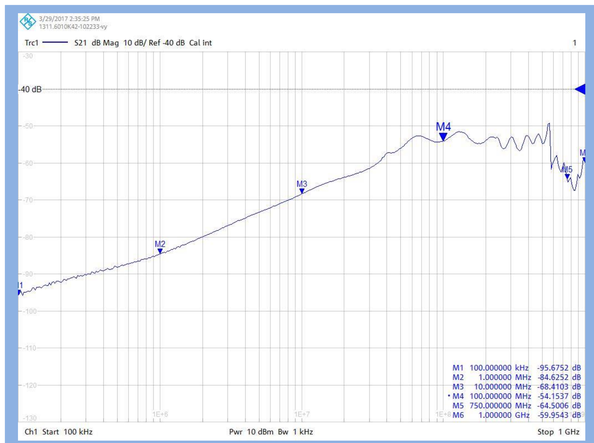
901プローブ周波数特性
