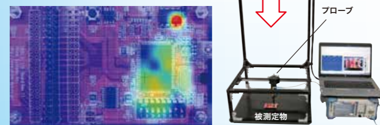
WM9500 alpha LTとプローブガイドにより、電装基板や電装ユニットの三次元電磁界ノイズ測定及び可視化が可能
