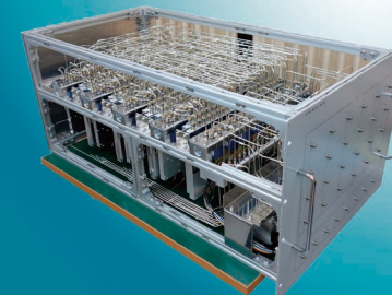
マトリックス・スイッチボックス
